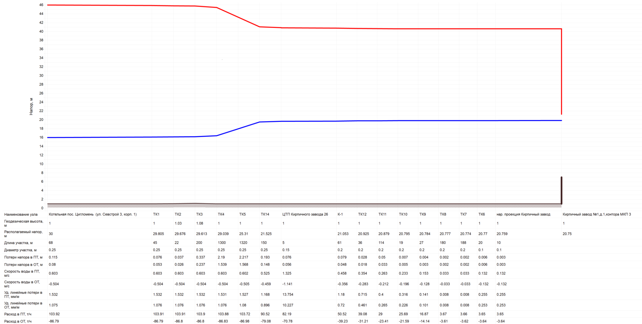
Рисунок 3.29 Существующий гидравлический режим тепловых сетей от котельной пос. Цигломень, ул. Севстрой 3, корп. 1
