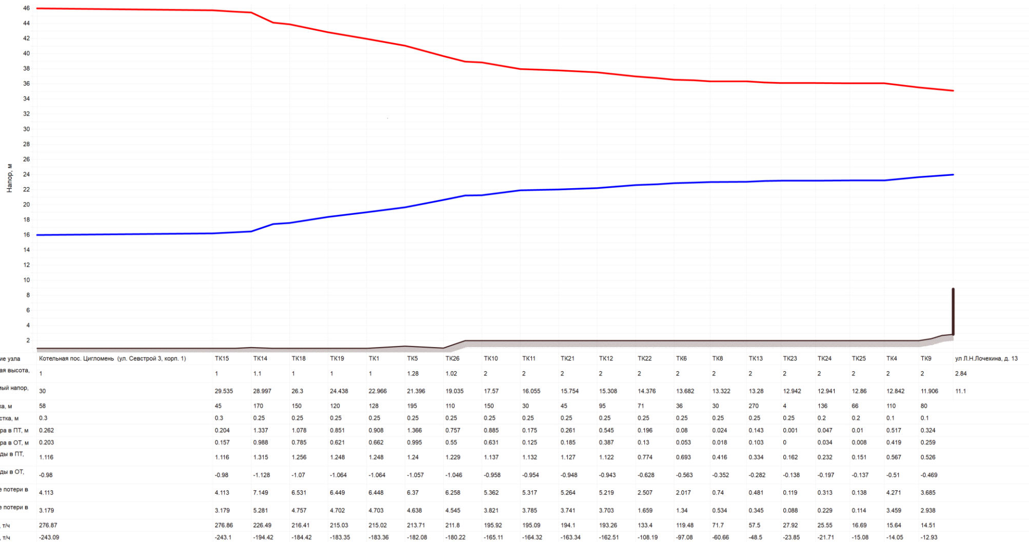
Рисунок 3.30 Существующий гидравлический режим тепловых сетей от котельной пос. Цигломень, ул. Севстрой 3, корп. 1
