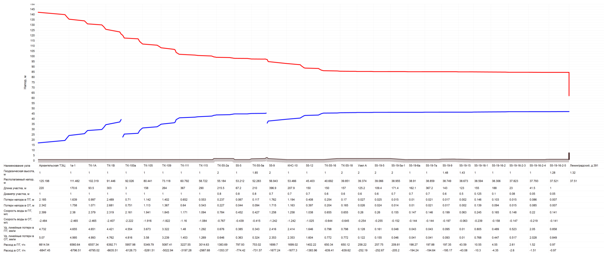
Рисунок 3.26 Существующий гидравлический режим тепловых сетей от Архангельской ТЭЦ
