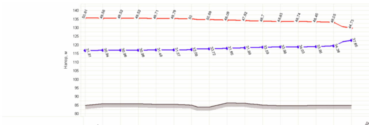
Рисунок 3.25 Пример пьезометрического графика
